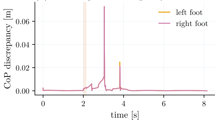
(d) contact-point discrepancy
