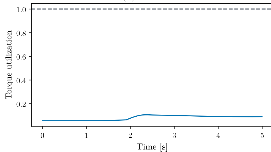
(d) Actuation
