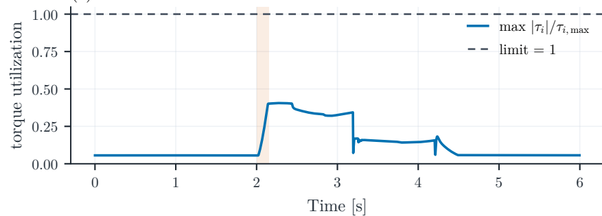
(e) actuator limit
