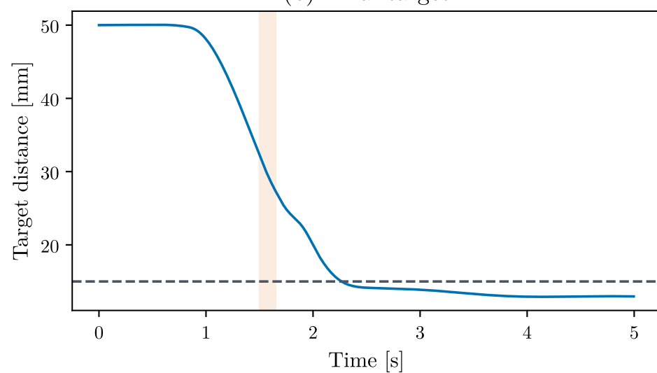
(d) Actuation
