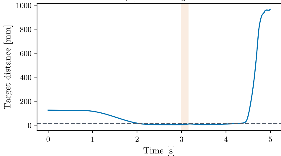
(d) Actuation
