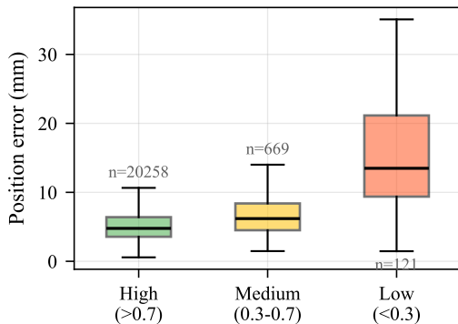
(d) Error by detection confidence
