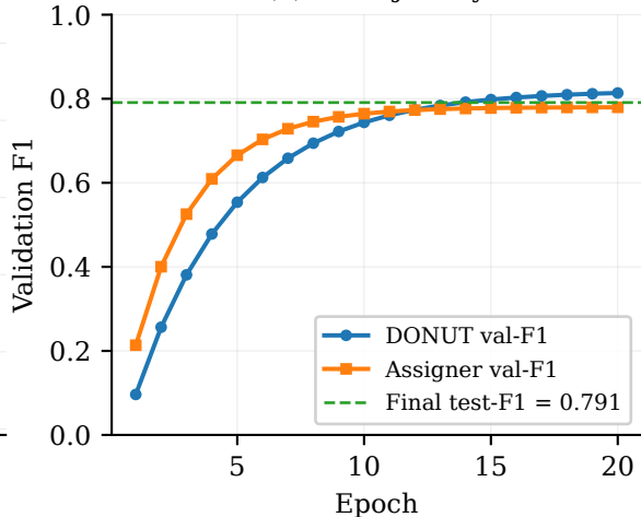
(b) F1 trajectory
