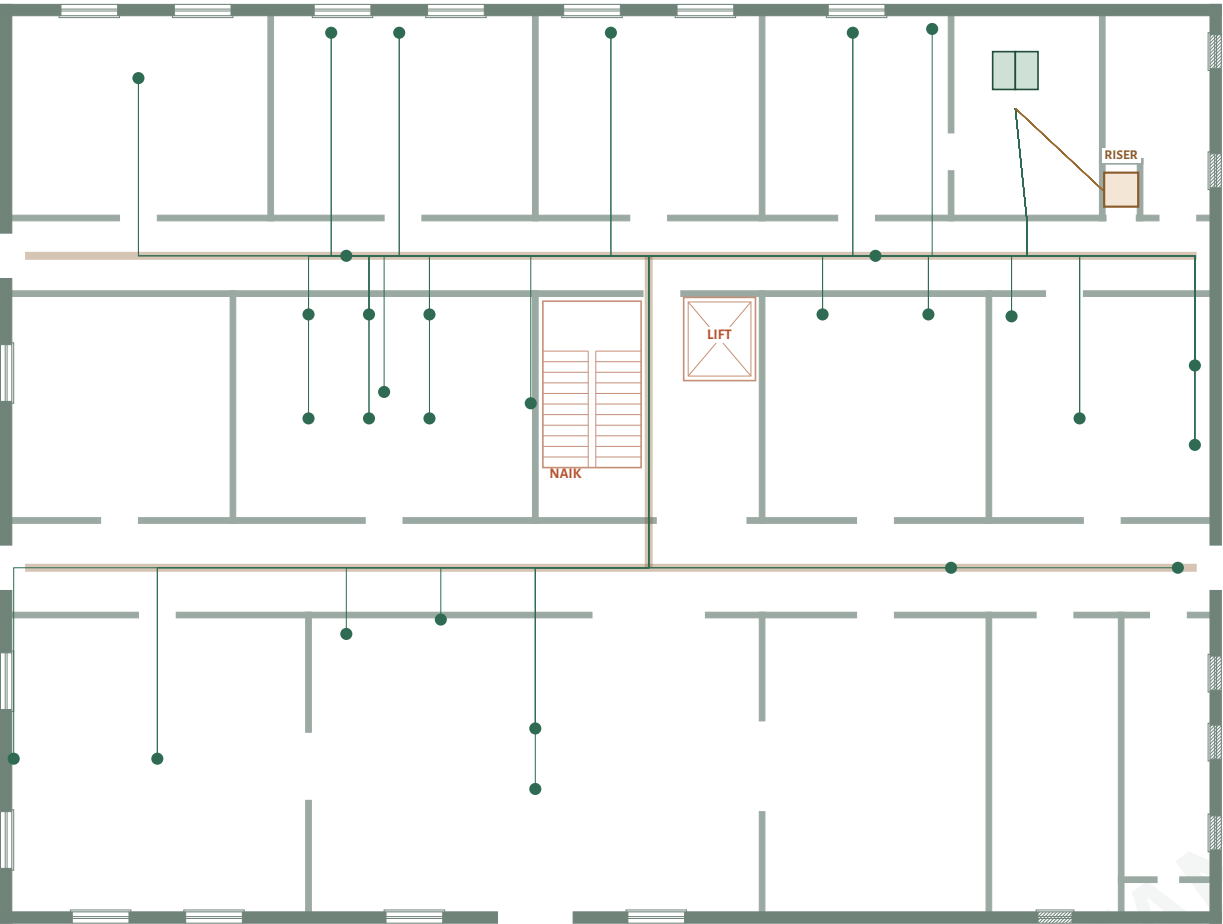
JALUR KABEL L1 1:200 - tray +3,2 m
