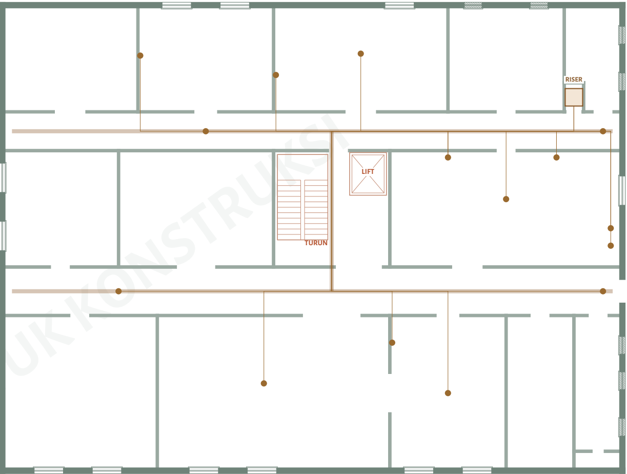
JALUR KABEL L2 1:200 - tray +3,2 m
