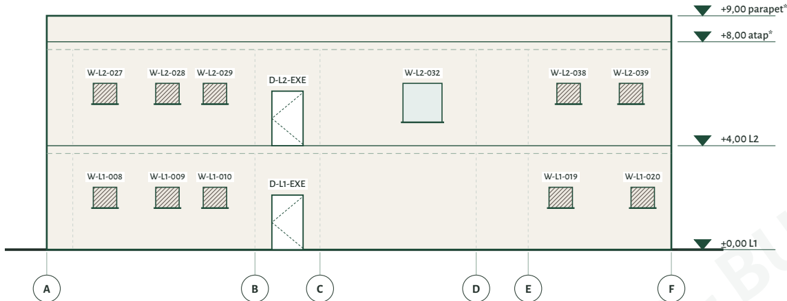
TAMPAK TIMUR 1:200
