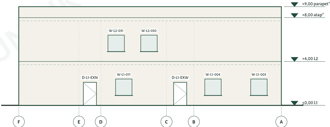
TAMPAK BARAT 1:200
