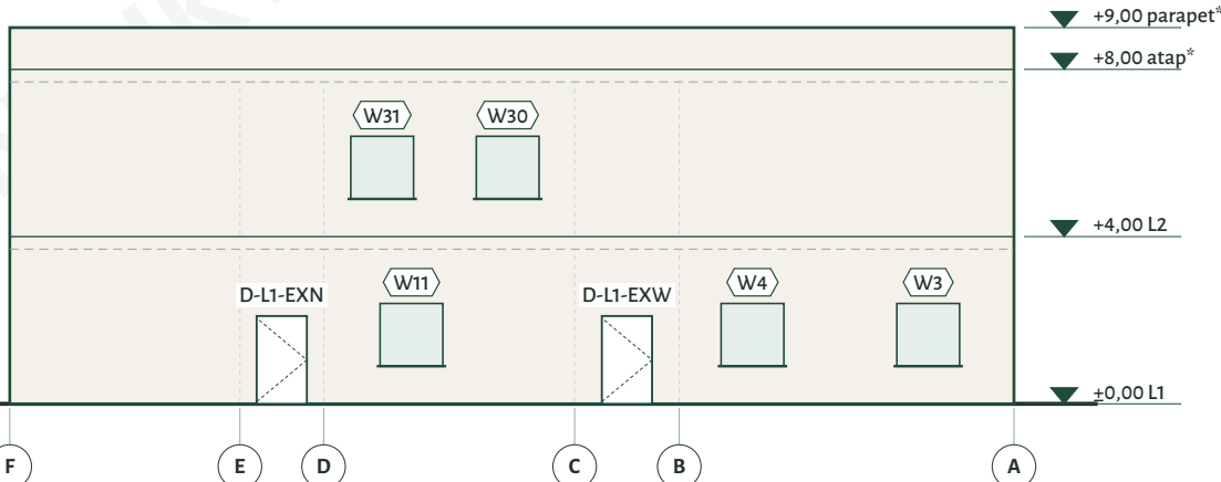
TAMPAK BARAT 1:200
