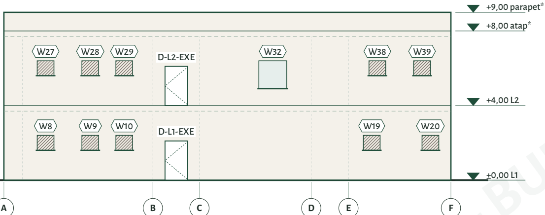
TAMPAK TIMUR 1:200
