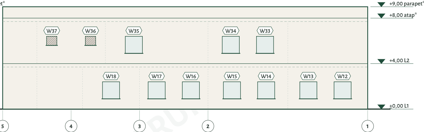
TAMPAK UTARA 1:200
