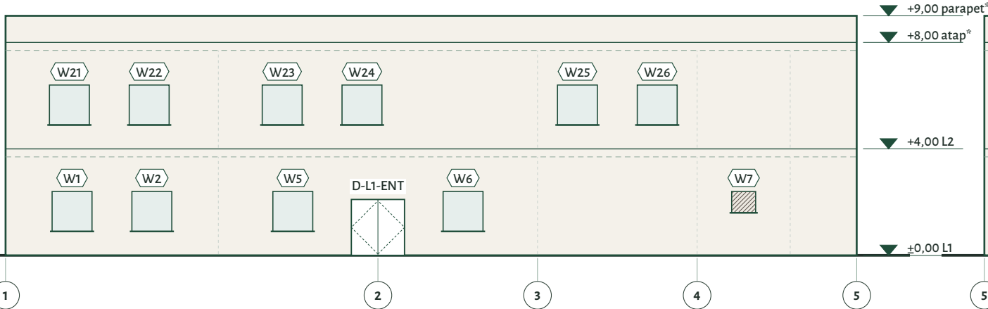
TAMPAK SELATAN 1:200
