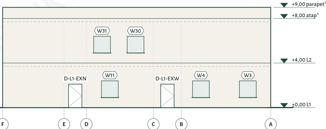
TAMPAK BARAT 1:200
