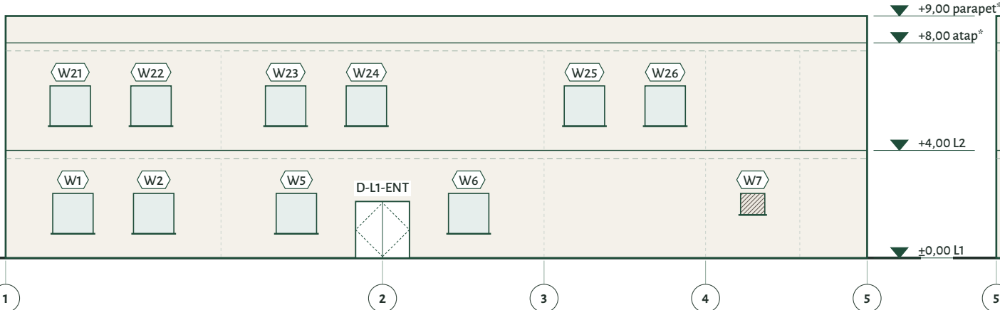
TAMPAK SELATAN 1:200
