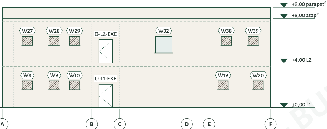
TAMPAK TIMUR 1:200
