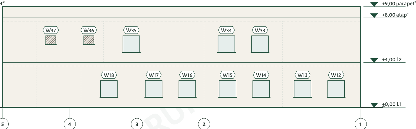
TAMPAK UTARA 1:200
