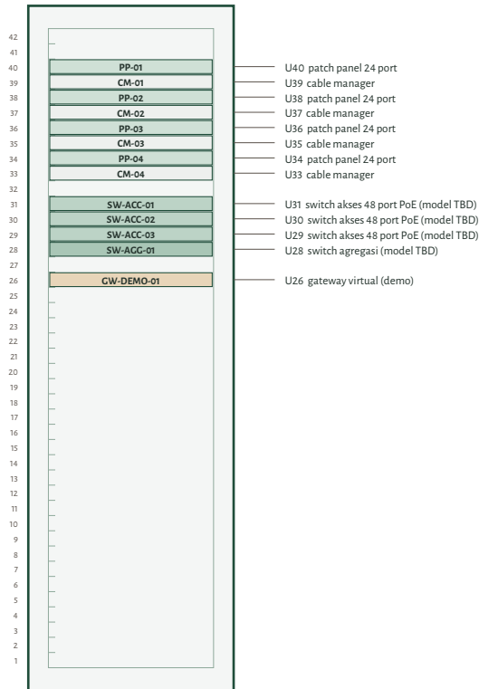
RK-L1-01 TAMPAK DEPAN 1:20 · L1-SERVER · 42U
