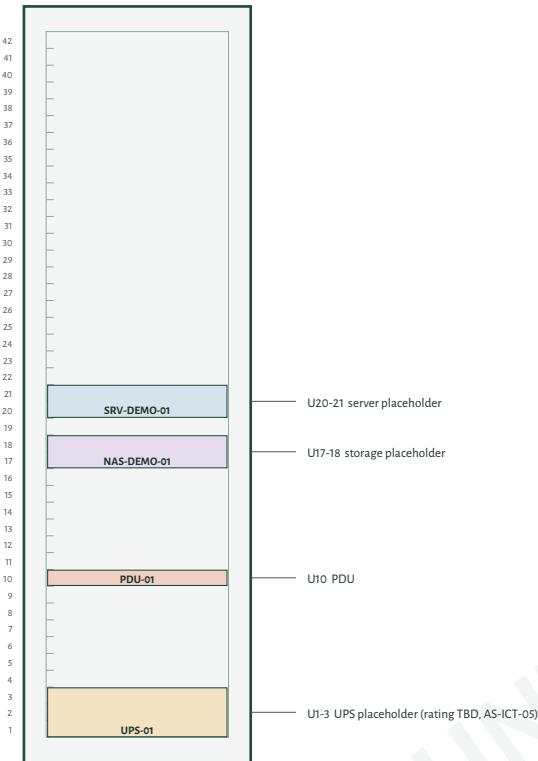
RK-L1-02 TAMPAK DEPAN 1:20 · L1-SERVER · 42U
