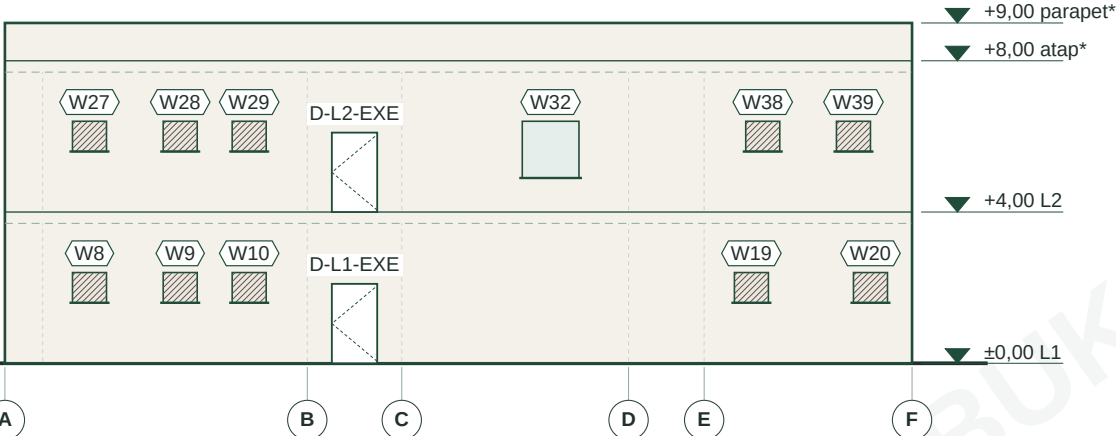
TAMPAK TIMUR 1:200
