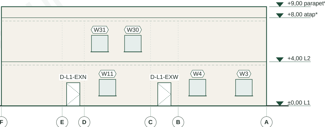
TAMPAK BARAT 1:200
