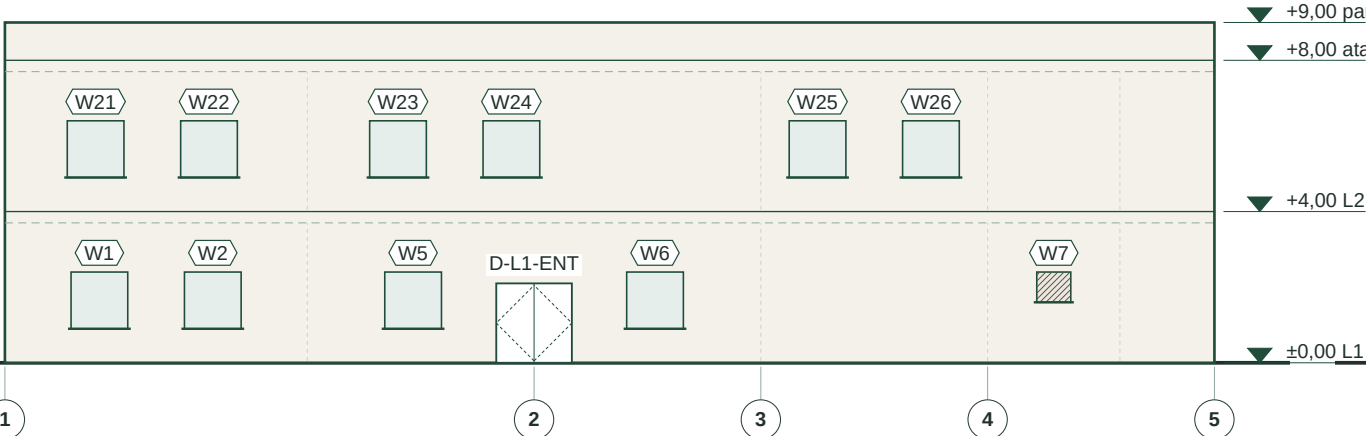
TAMPAK SELATAN 1:200
