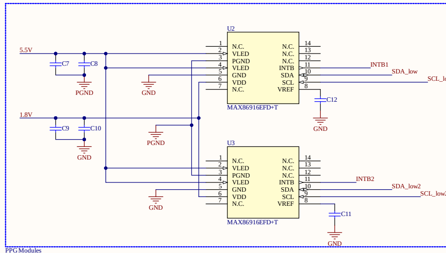
PPG Modules
