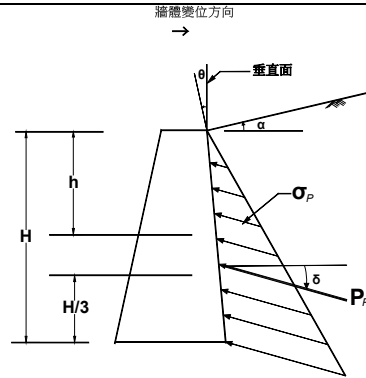
圖 6-5 被動土壓力圖
