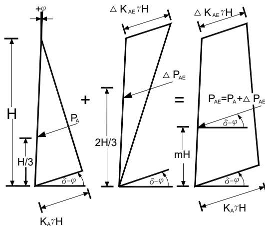
圖 6-6 動態主動土壓力及幾何關係示意圖
