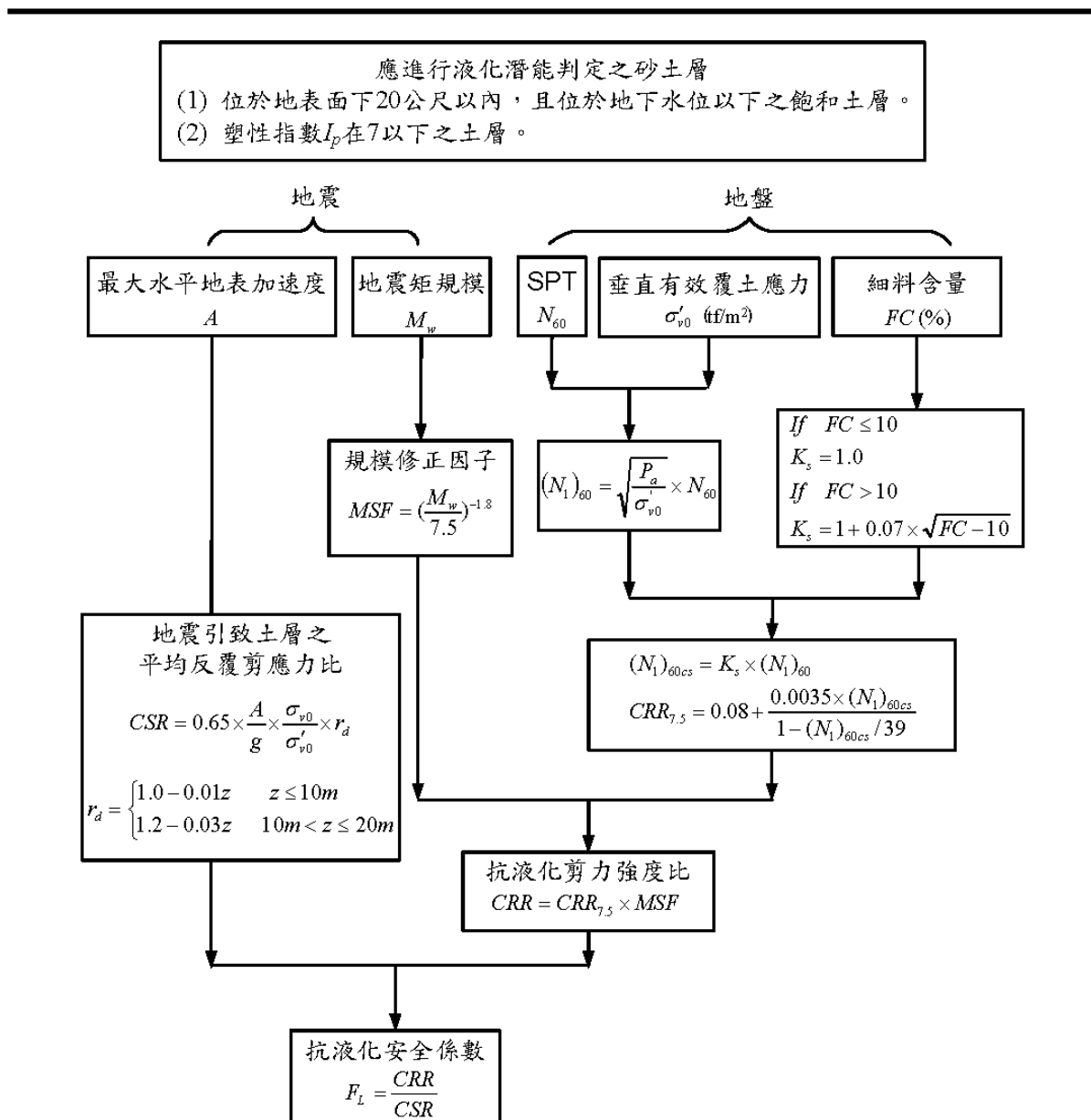
圖 6-16 雙曲線函數(HBF)液化評估法之計算流程
