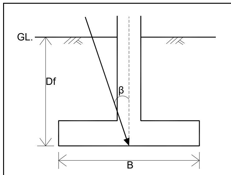
圖 6-1 淺基礎示意圖
