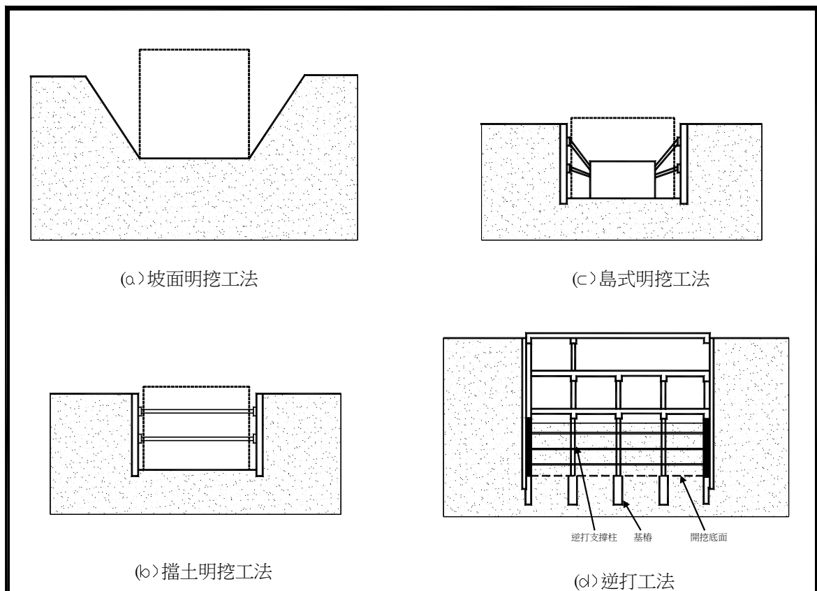
圖 6-14 開挖工法示意圖
