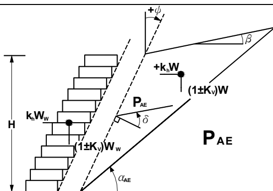
圖 6-4 主動土壓力圖
