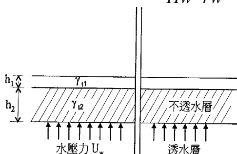
上舉水壓力檢討
