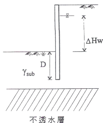
圖 6-13 砂湧檢討
