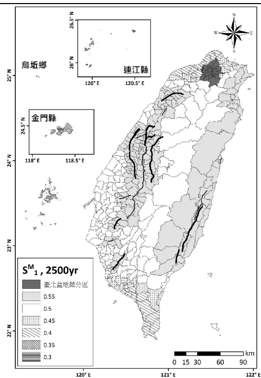
圖 5-4 基地短週期設計水平譜加速度係數 S_1^M 分布圖
