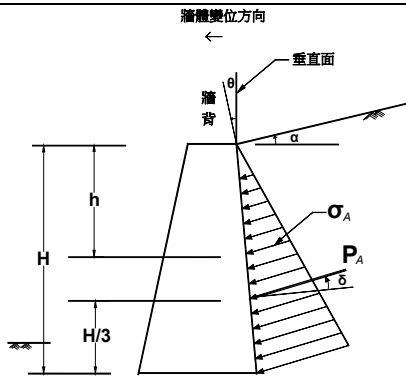
圖 6-4 主動土壓力圖
