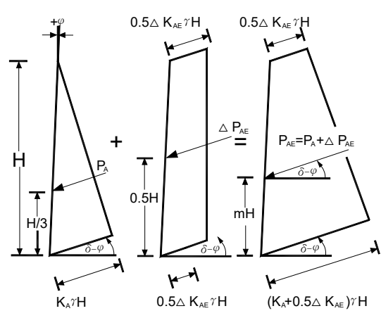
圖 6-7 動態主動土壓力之分布圖
