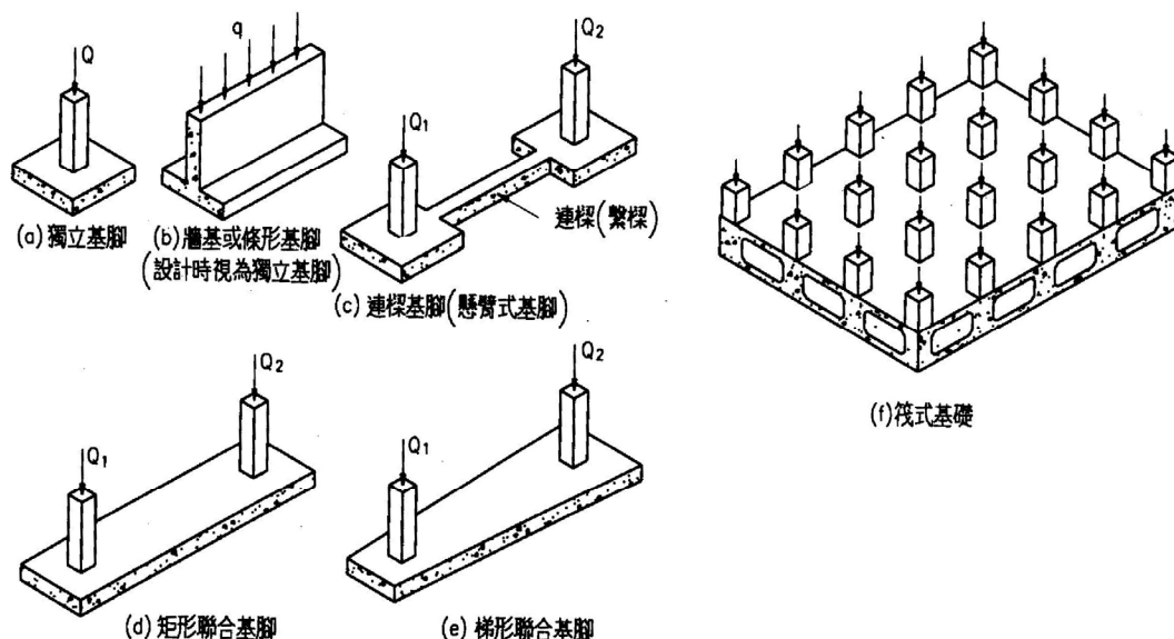
圖 6-3 基礎型式示意圖
