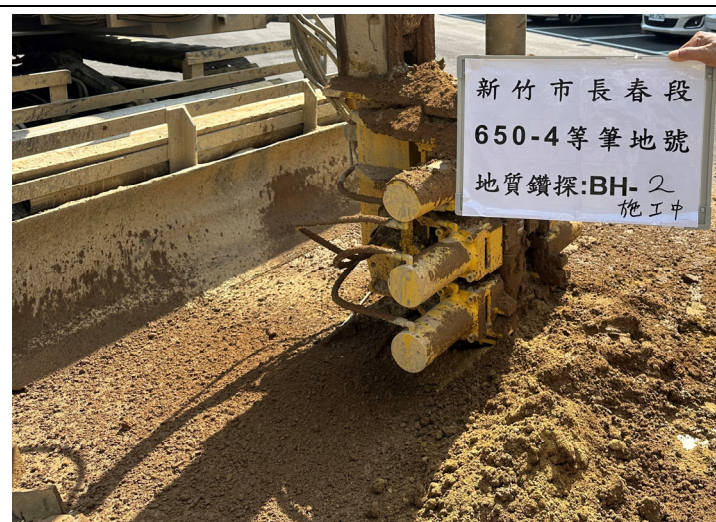
BH-2 施工中
