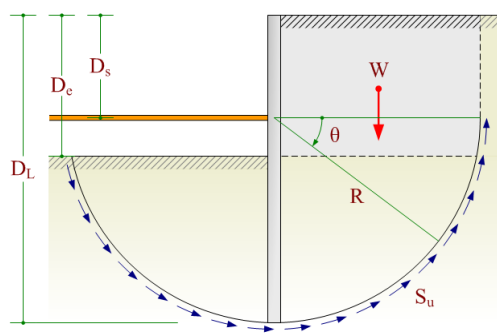
圖 6-11 開挖面隆起穩定分析
