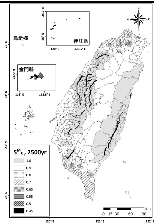
圖 5-3 基地短週期設計水平譜加速度係數 S_s^M 分布圖
