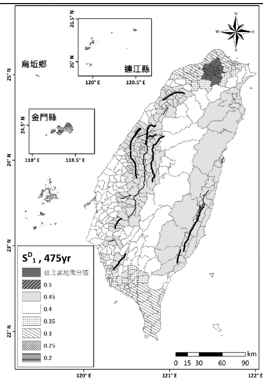
圖 5-2 基地一秒週期設計水平譜加速度係數 S_1^D 分布圖
