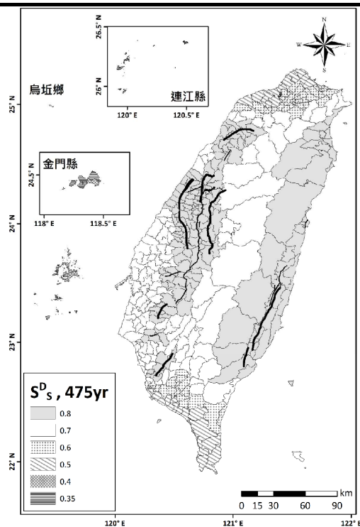
圖 5-1 基地短週期設計水平譜加速度係數 S_s^D 分布圖
