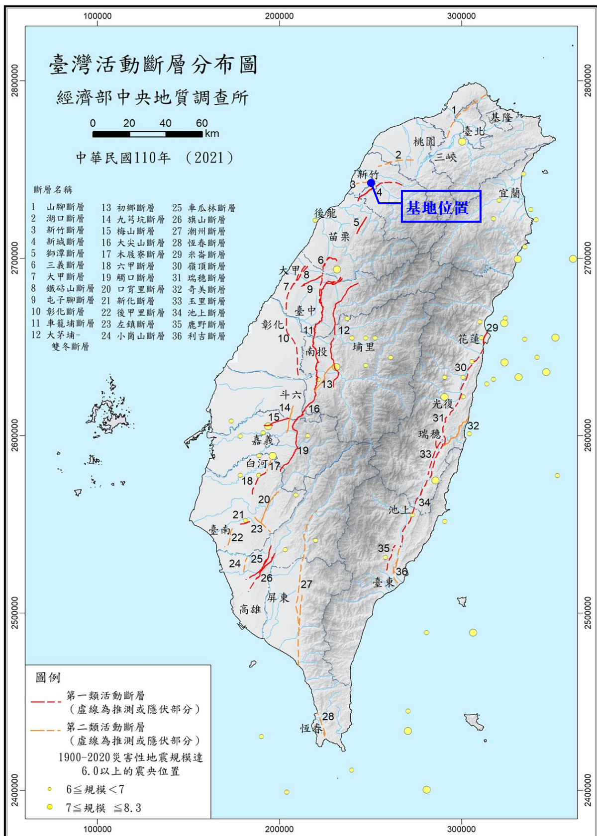
圖 3-2 臺灣活動斷層分布圖
