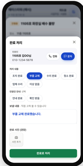
② 완료 처리 창 맨 위 전화 · 문자
