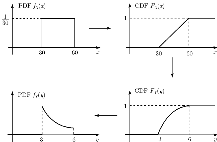
图 4.1 例 4.2 中 Y = 180/X 的概率密度函数的计算过程示意图. 箭头方向表示计算步骤
