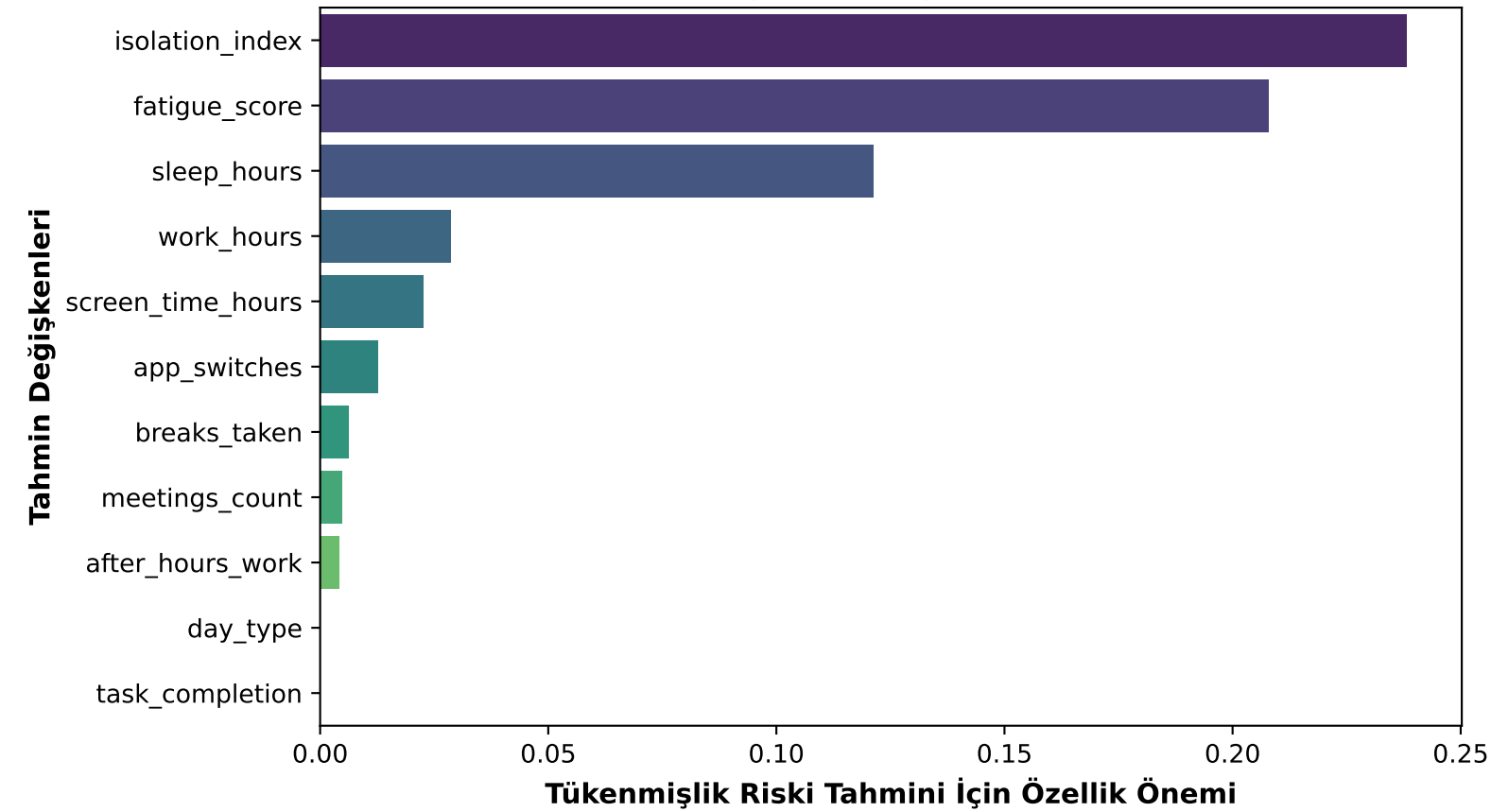
SVM
