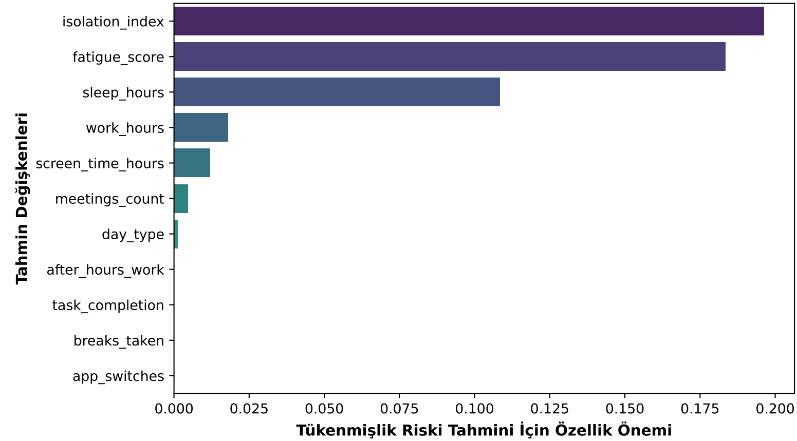
SVM
