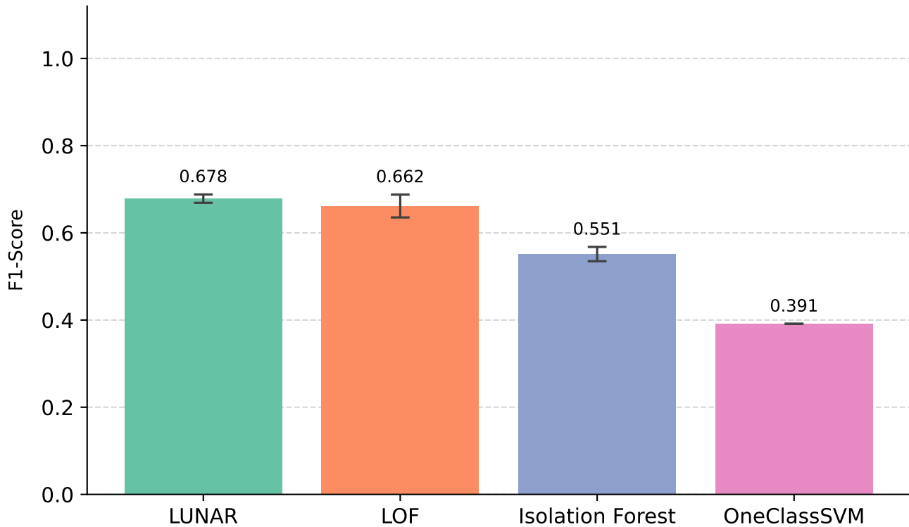
F1 modeli pojedynczych (próg standardowy) — CICIDS 2017
