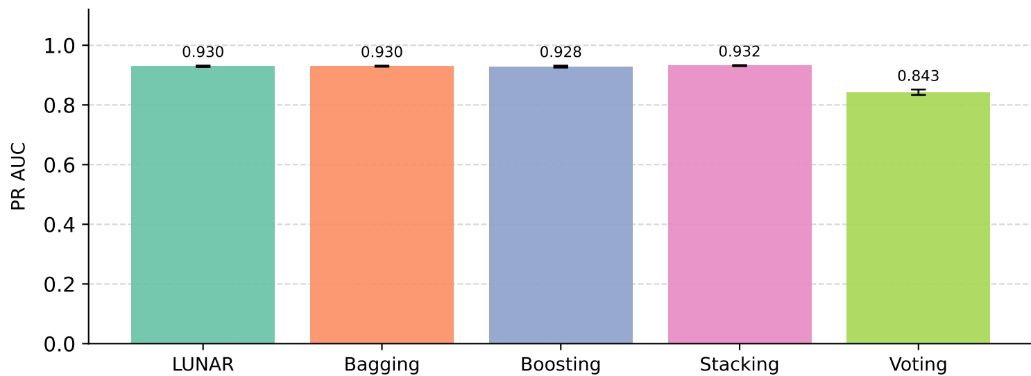
UNSW-NB15
