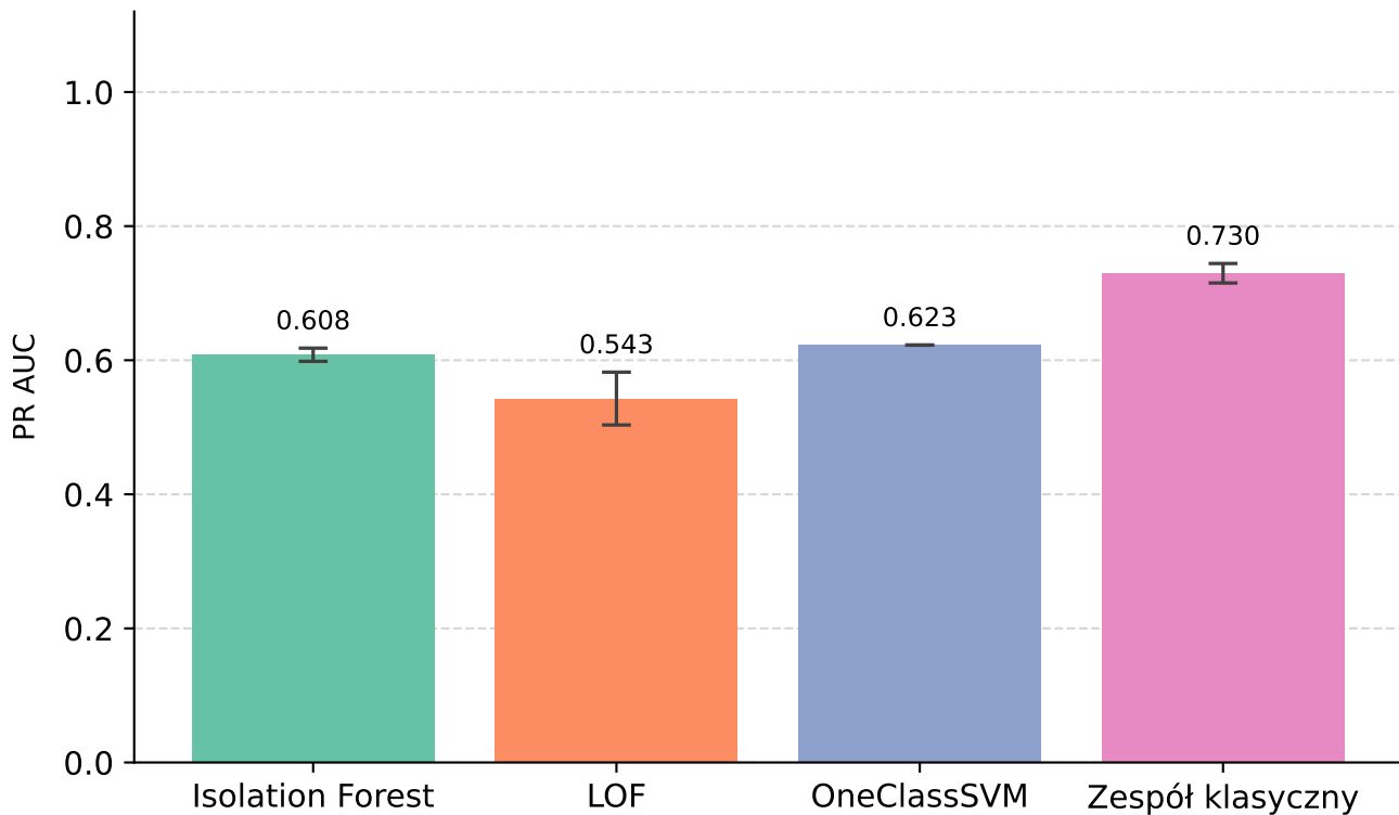
PR AUC: modele klasyczne pojedyncze vs zespół klasyczny — CICIDS 2017
