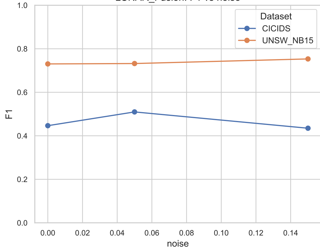
LUNAR_Fusion: F1 vs noise
