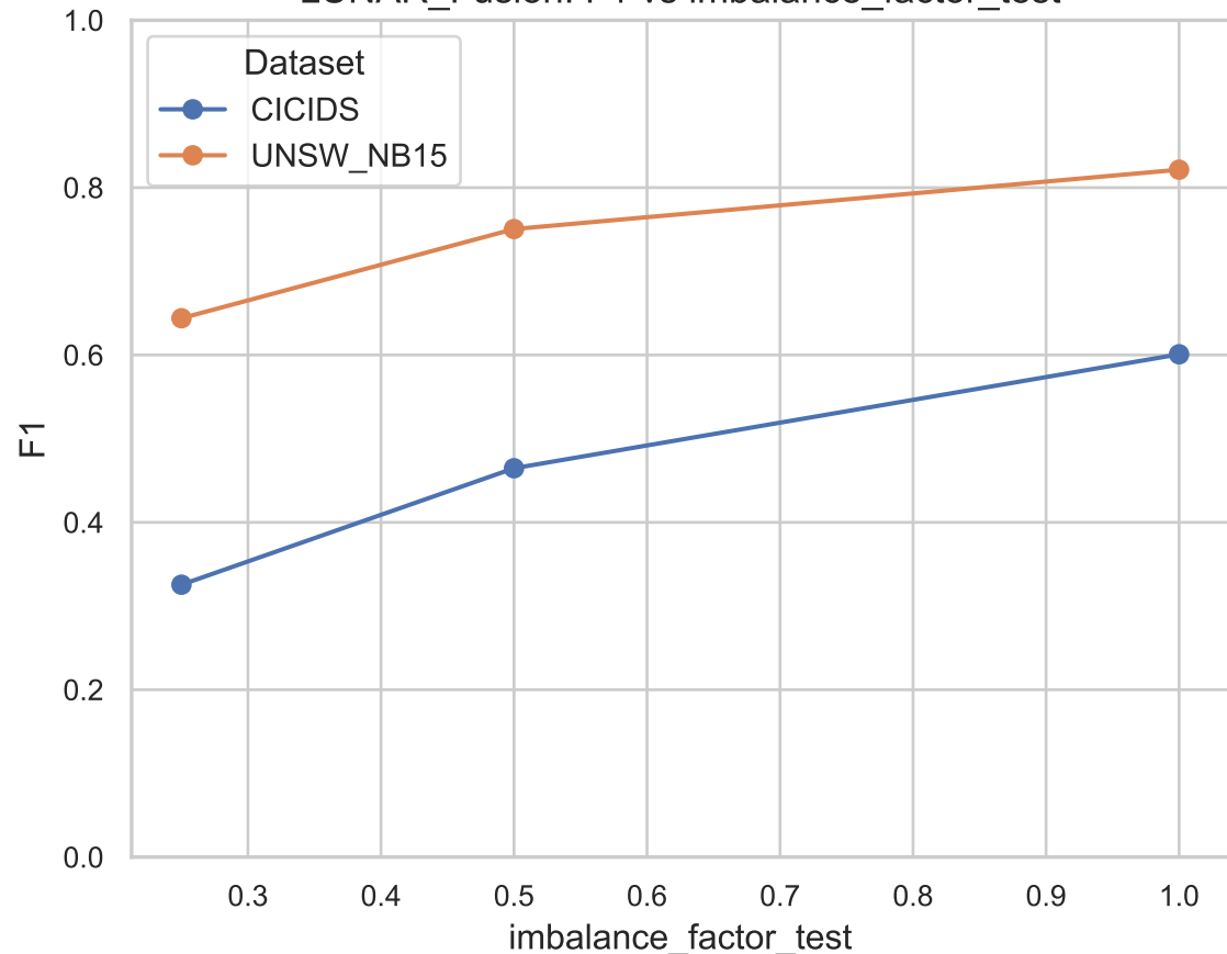
LUNAR_Fusion: F1 vs imbalance_factor_test
