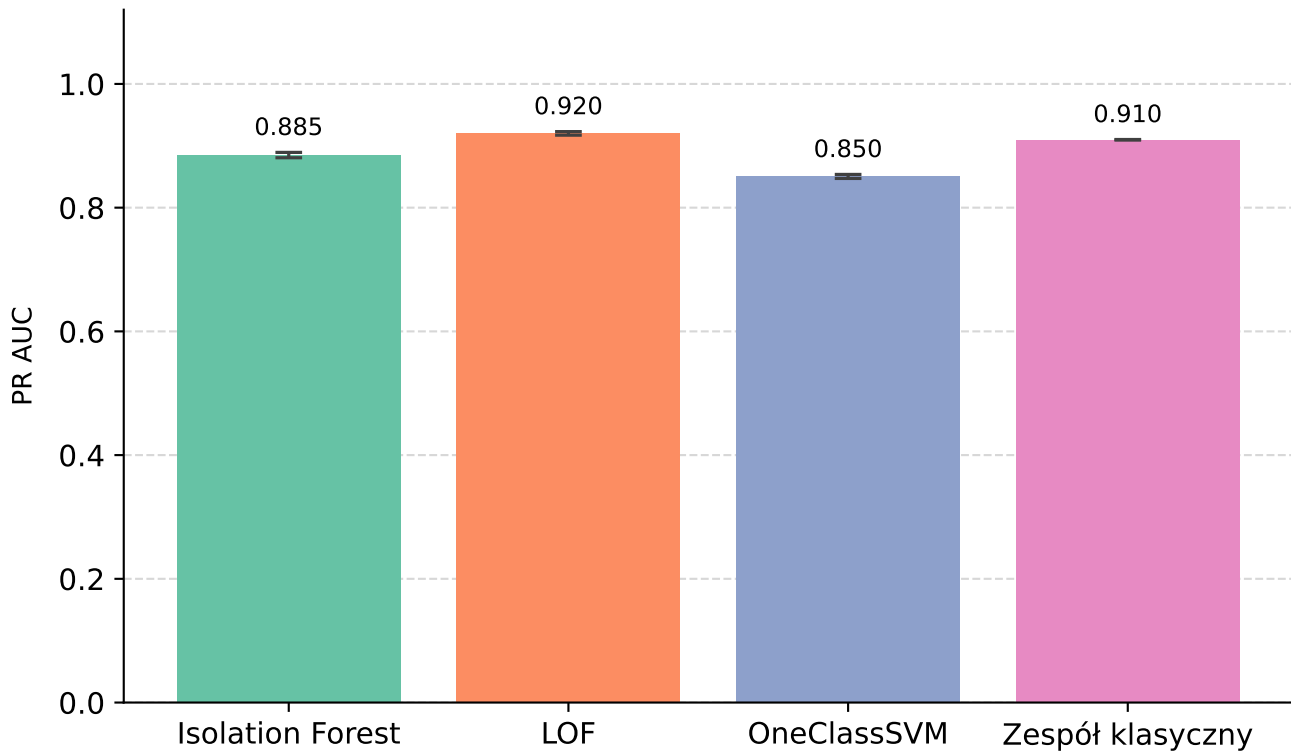
PR AUC: modele klasyczne pojedyncze vs zespół klasyczny — UNSW-NB15
