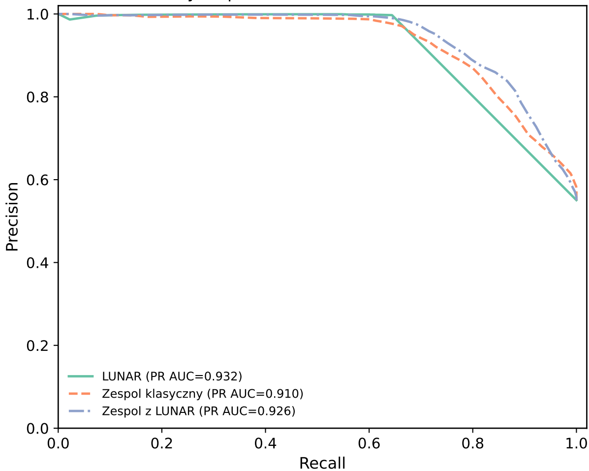
Krzywe precision-recall -- UNSW-NB15
