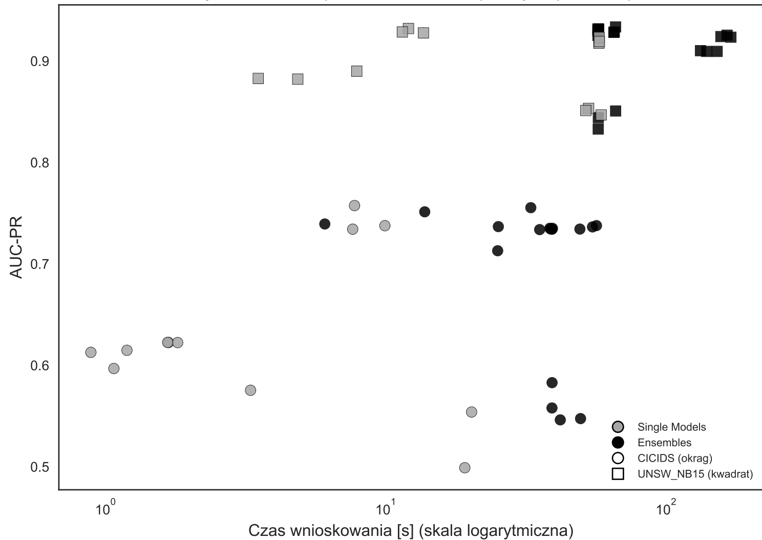
Wykres 5. Koszt (czas wnioskowania) vs zysk (AUC-PR)
