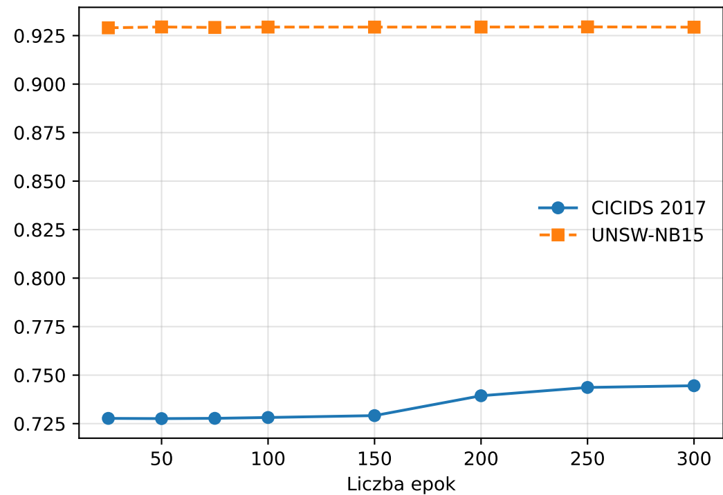
PR AUC
