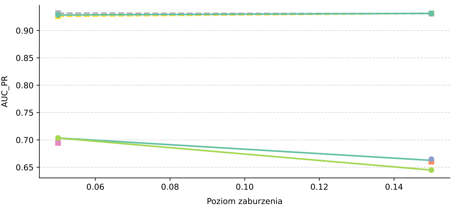
Metryka: AUC_PR
