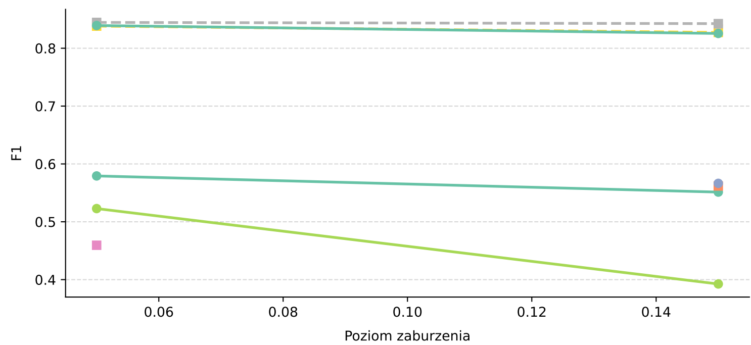
Metryka: F1
