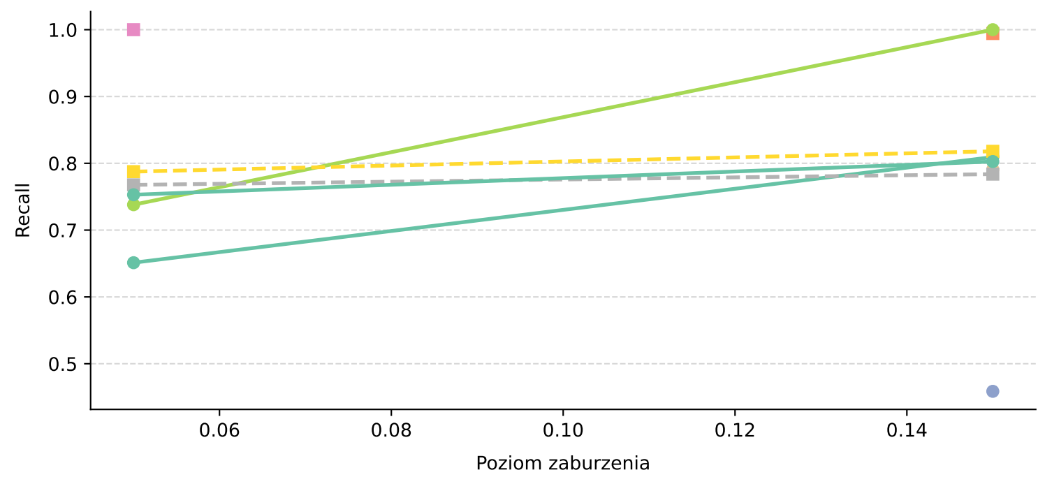
Metryka: Recall
