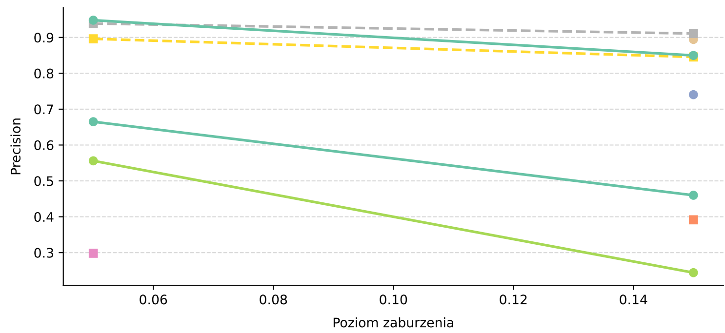
Metryka: Precision
