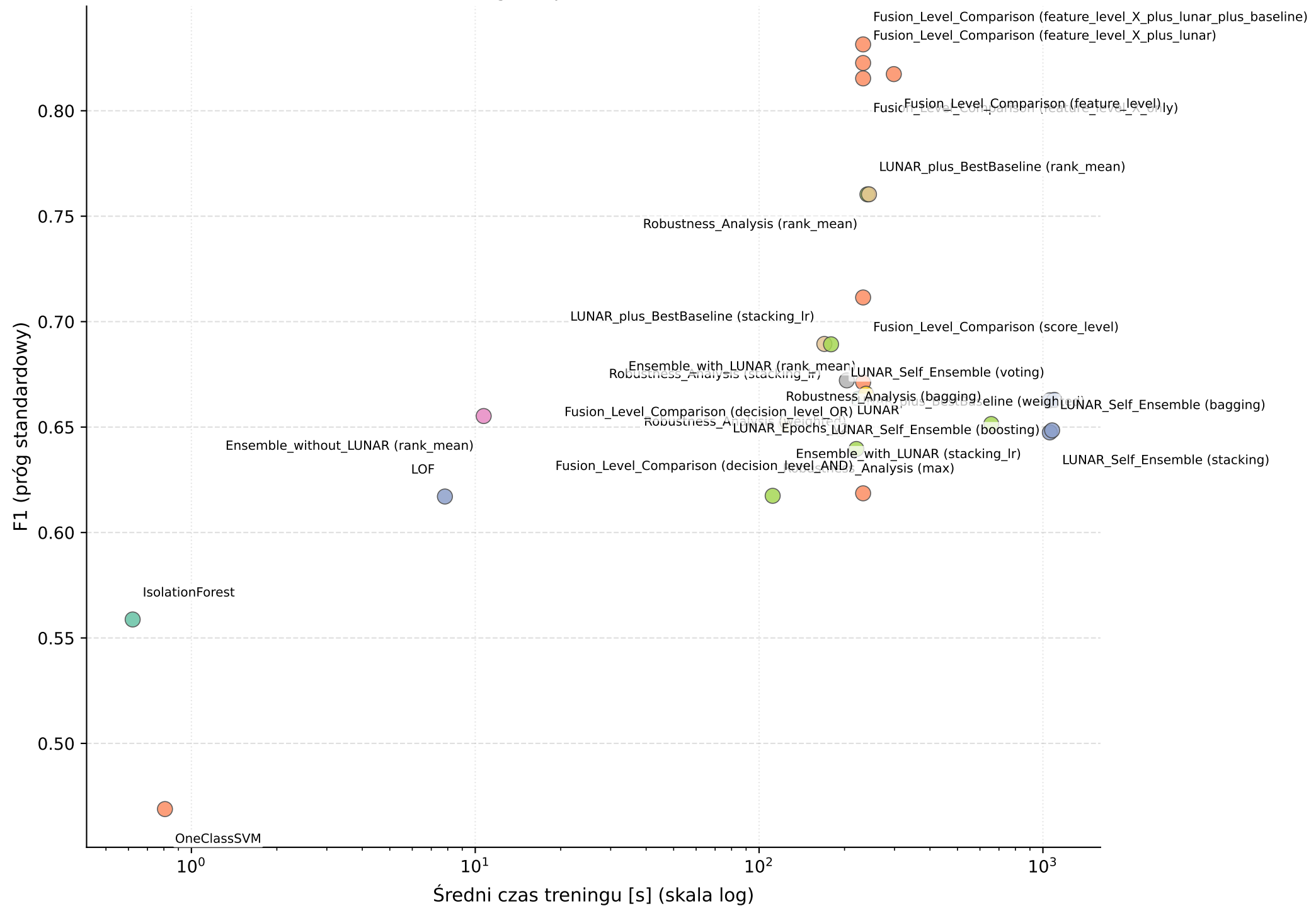
Koszt treningu vs jakość (F1) - CICIDS 2017
