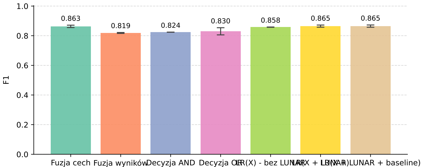
UNSW-NB15
