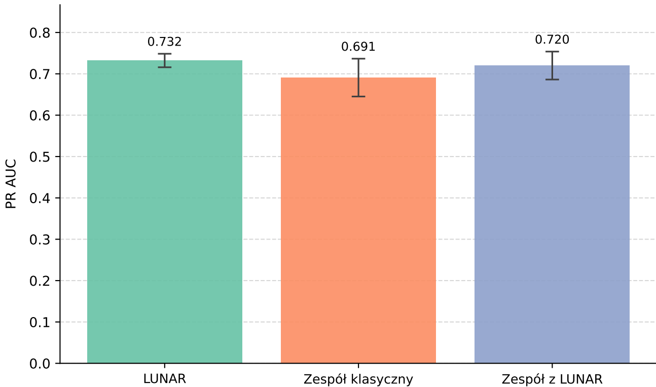
Wkład LUNAR w zespole (PR AUC) - CICIDS 2017
