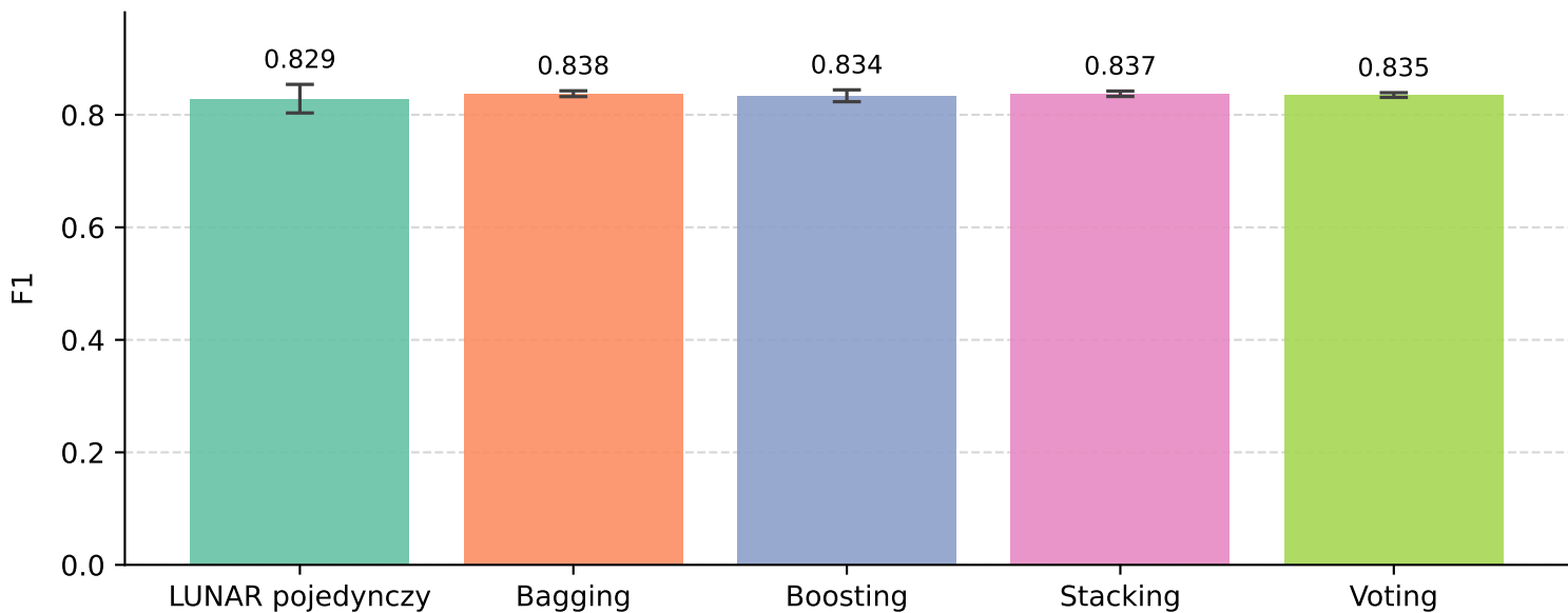
UNSW-NB15
