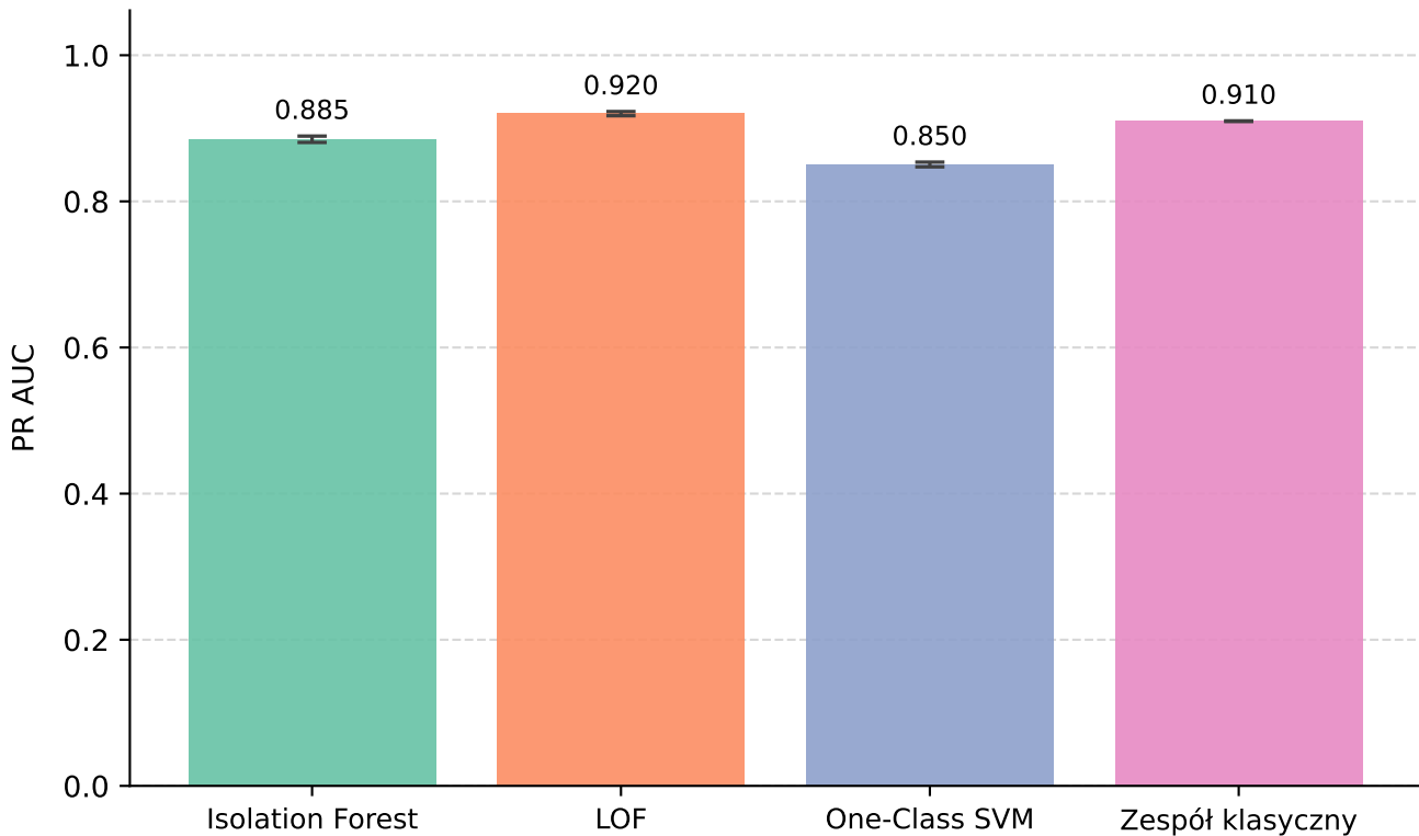
PR AUC modeli klasycznych i zespołu klasycznego - UNSW-NB15
