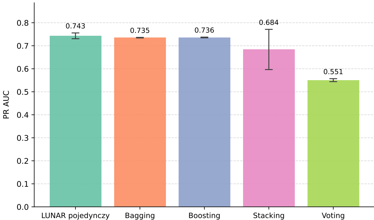
PR AUC: LUNAR pojedynczy i zespoły homogeniczne - CICIDS 2017
