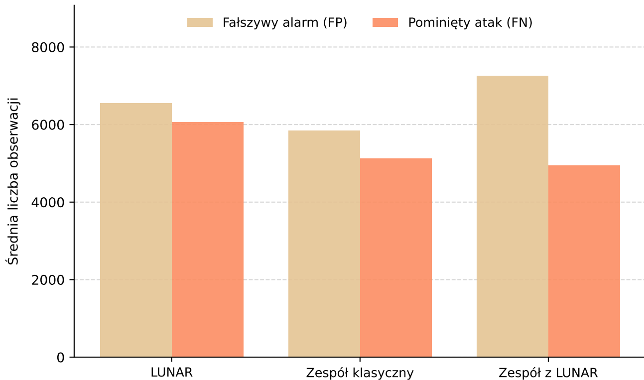
Liczba fałszywych alarmów (FP) i pominiętych ataków (FN) — CICIDS 2017
