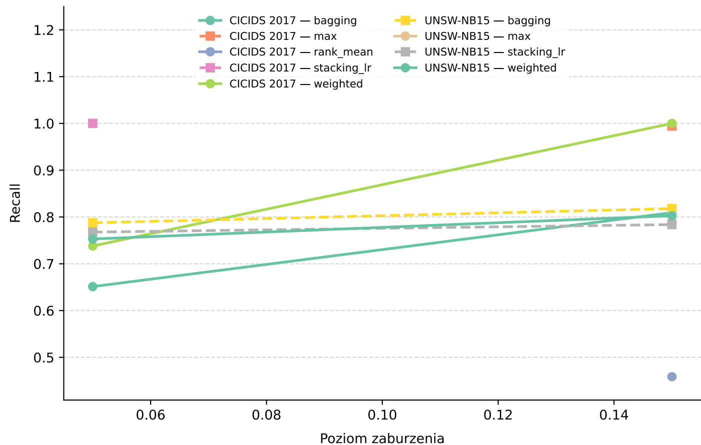
Recall — scenariusz: Szum
