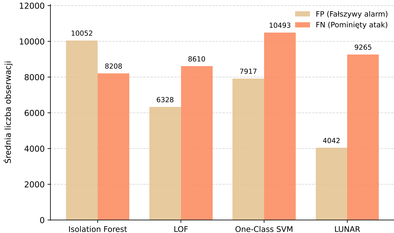
Fałszywe alarmy (FP) i pominięte ataki (FN) — UNSW-NB15
