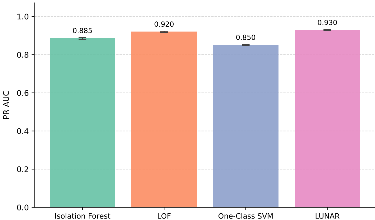
Porównanie PR AUC modeli pojedynczych - UNSW-NB15
