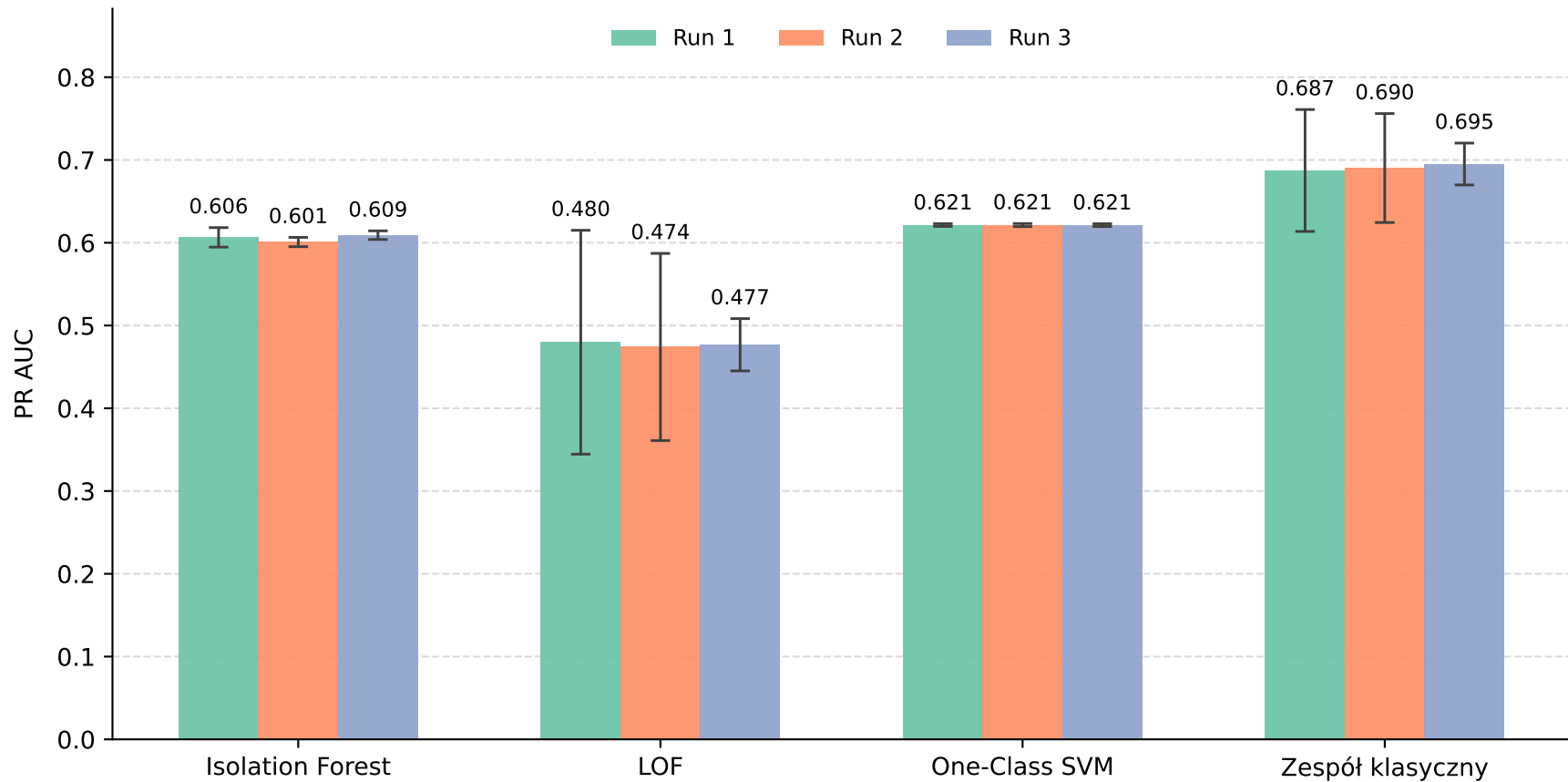
PR AUC modeli klasycznych i zespołu klasycznego — CICIDS 2017
