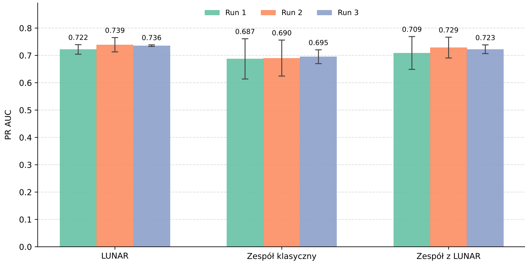
Wkład LUNAR w zespole (PR AUC) — CICIDS 2017
