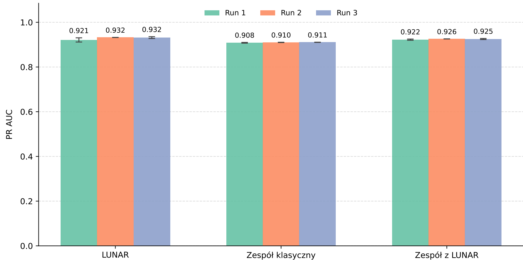
Wkład LUNAR w zespole (PR AUC) — UNSW-NB15
