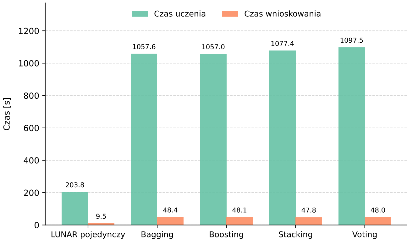
Koszt uczenia i wnioskowania: LUNAR vs zespoły — CICIDS 2017
