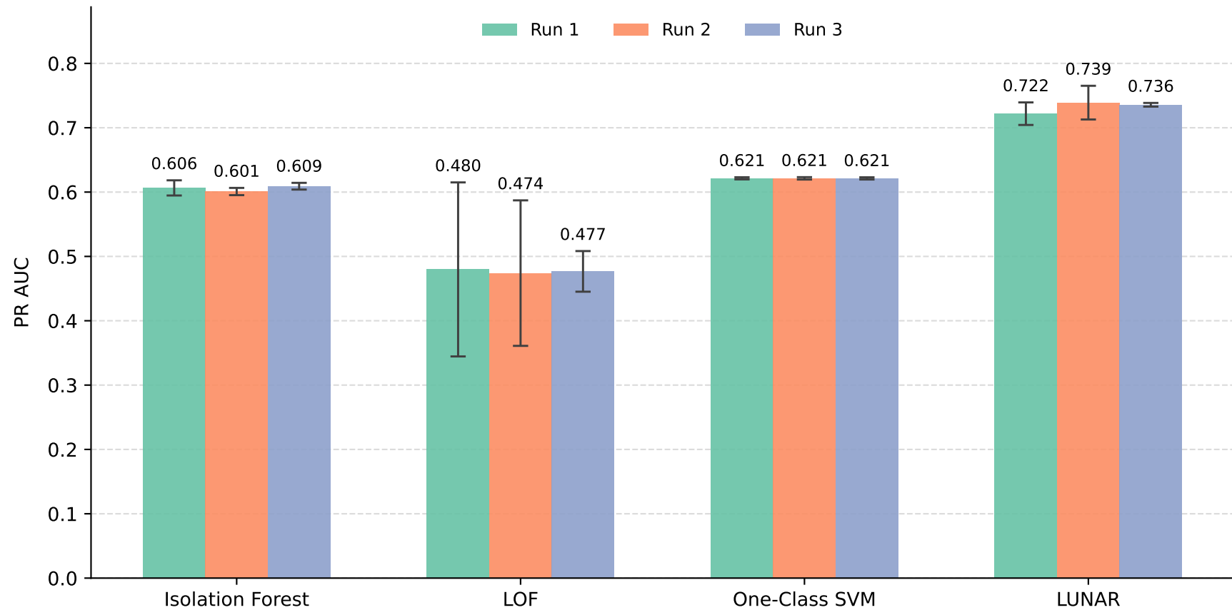
Porównanie PR AUC modeli pojedynczych — CICIDS 2017
