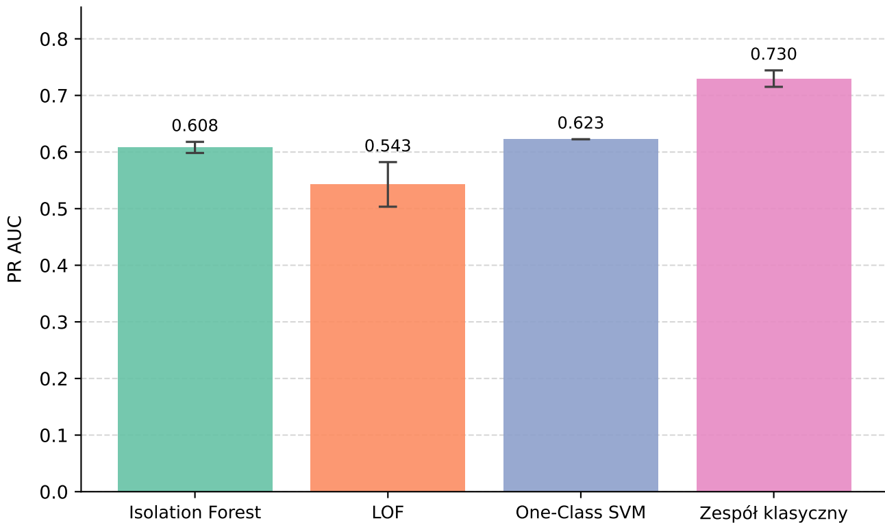
PR AUC modeli klasycznych i zespołu klasycznego - CICIDS 2017
