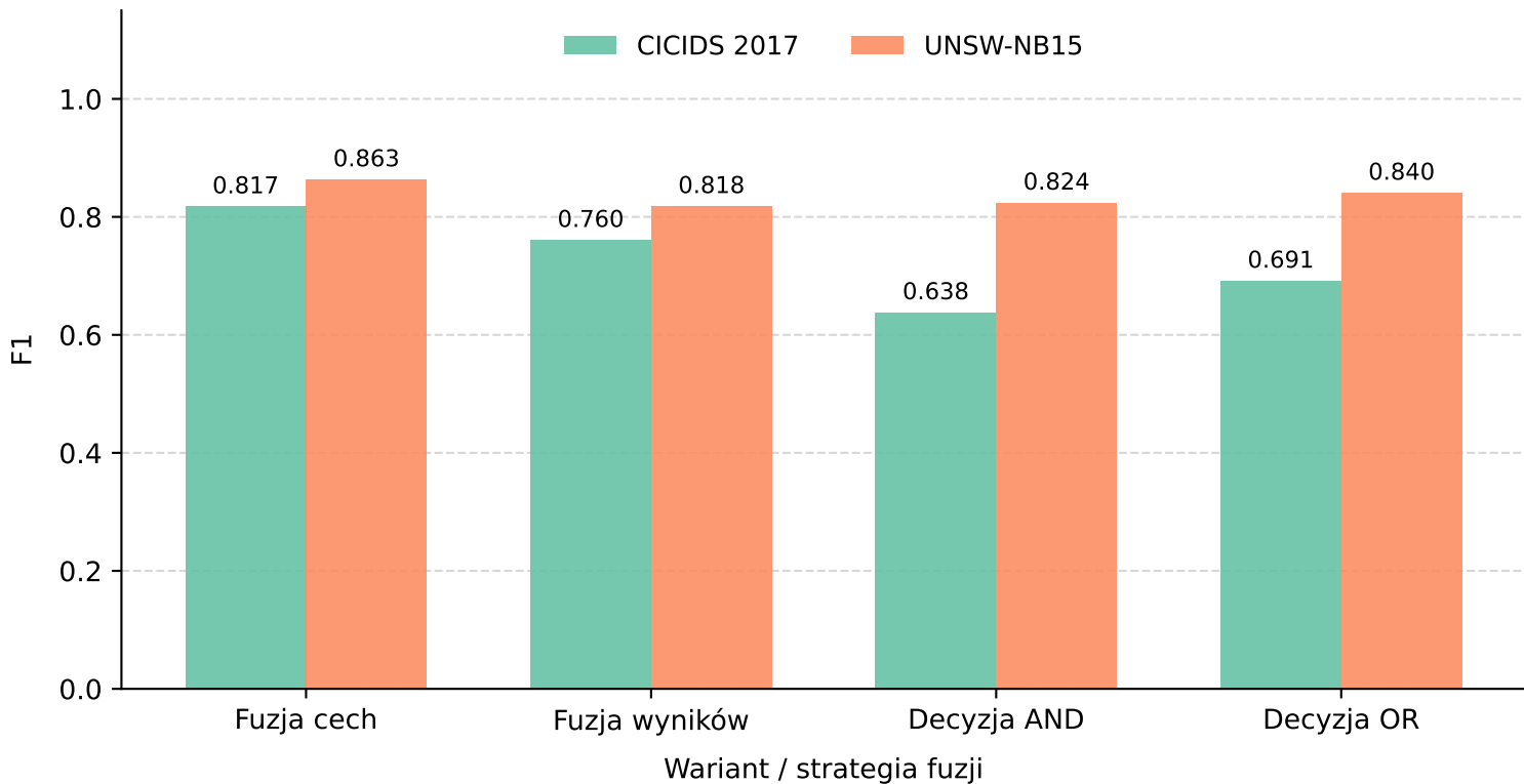
F1 przy progu standardowym — wszystkie warianty fuzji
