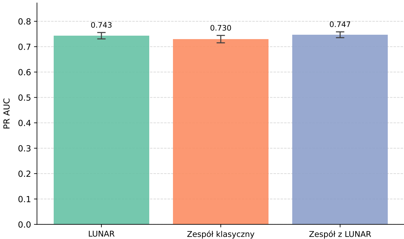
Wkład LUNAR ponad agregację klasyczną - CICIDS 2017
