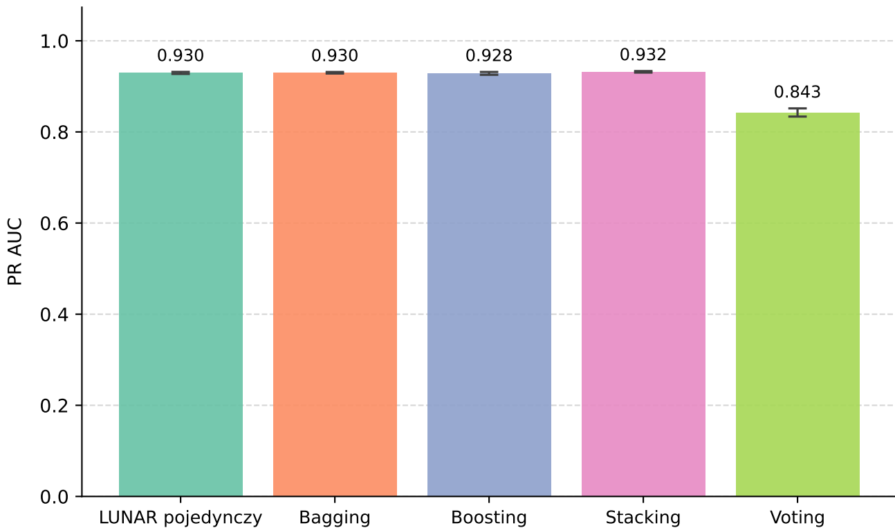
PR AUC: LUNAR pojedynczy i zespoły homogeniczne - UNSW-NB15
