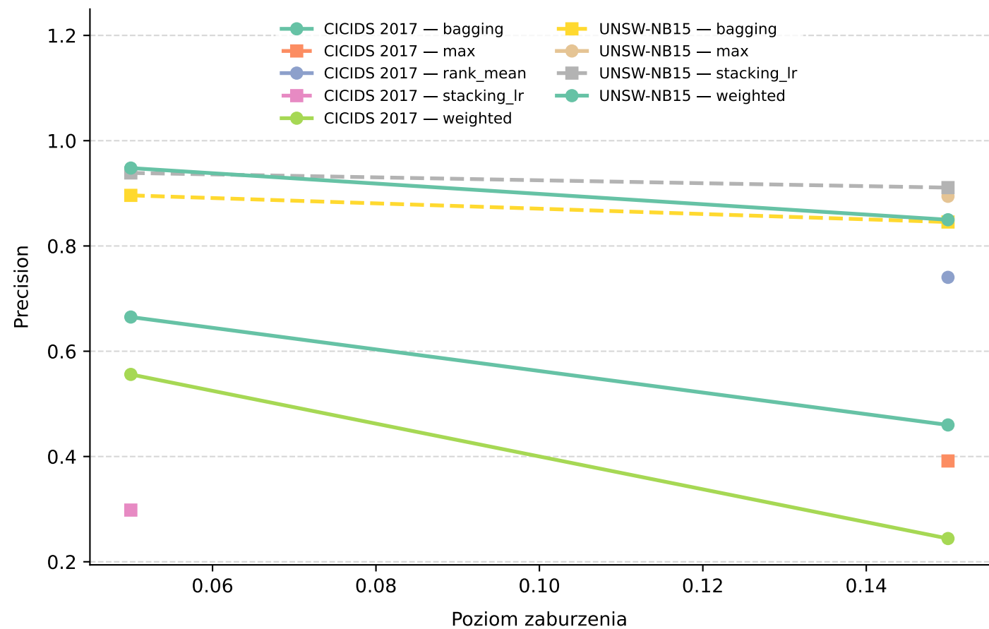
Precision — scenariusz: Szum
