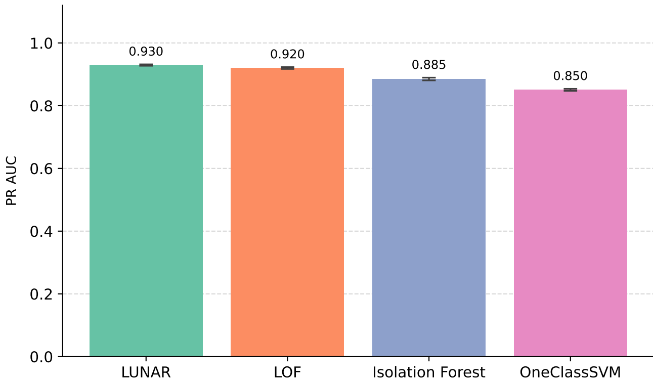
PR AUC modeli pojedynczych - UNSW-NB15
