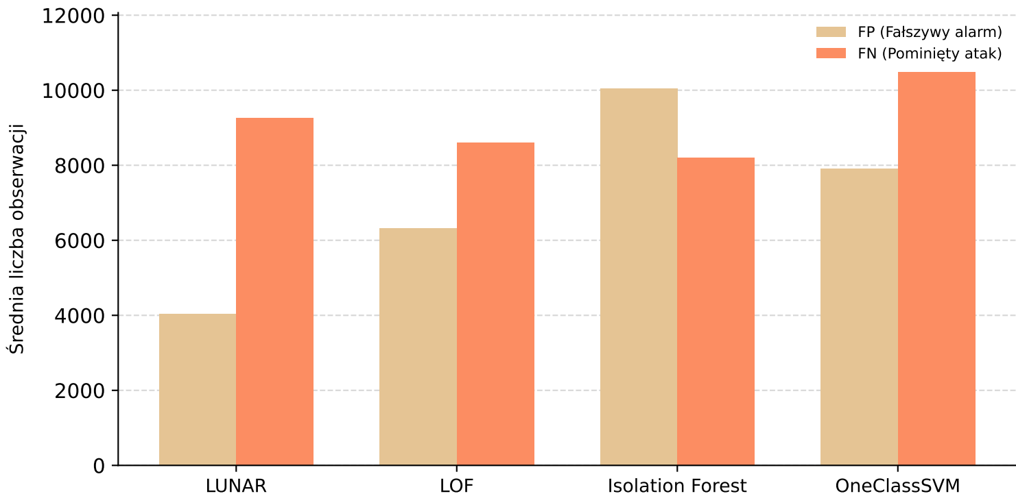
UNSW-NB15
